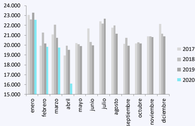
Evolución mensual de la demanda de electricidad, Enero 2017 - abril 2020. Sistema peninsular. GWh
